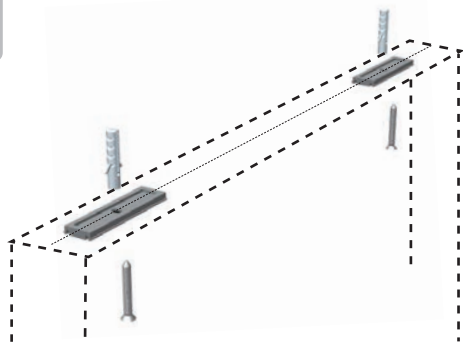
Fissaggio laterale
